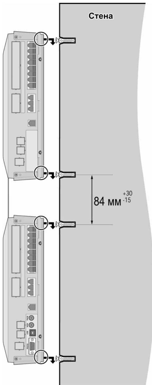
Рис. 3.3.3.16 Настенный монтаж блоков
