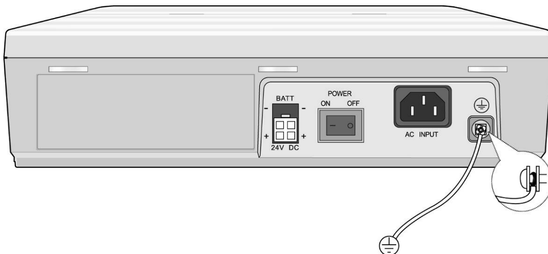
Рис. 3.2.5 Заземление корпуса
