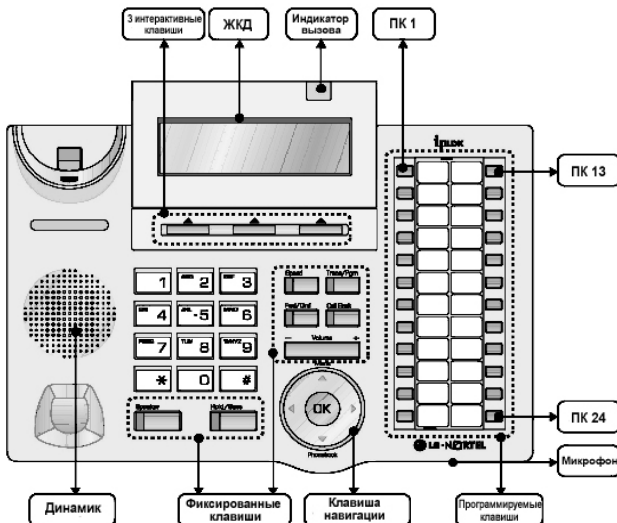
Рис. 6.2.1.1 Описание клавиш цифрового аппарата LDP-7024D
