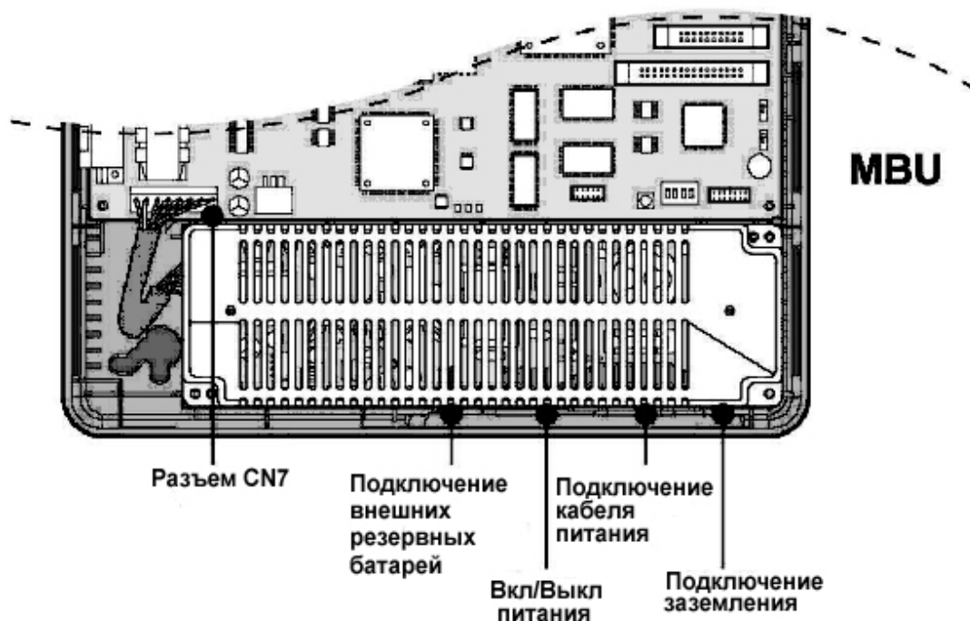
Рис. 3.2.4 Установка блока питания
