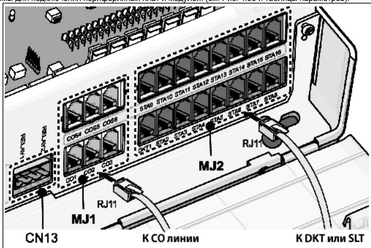
Рис. 4.36 Подключение
