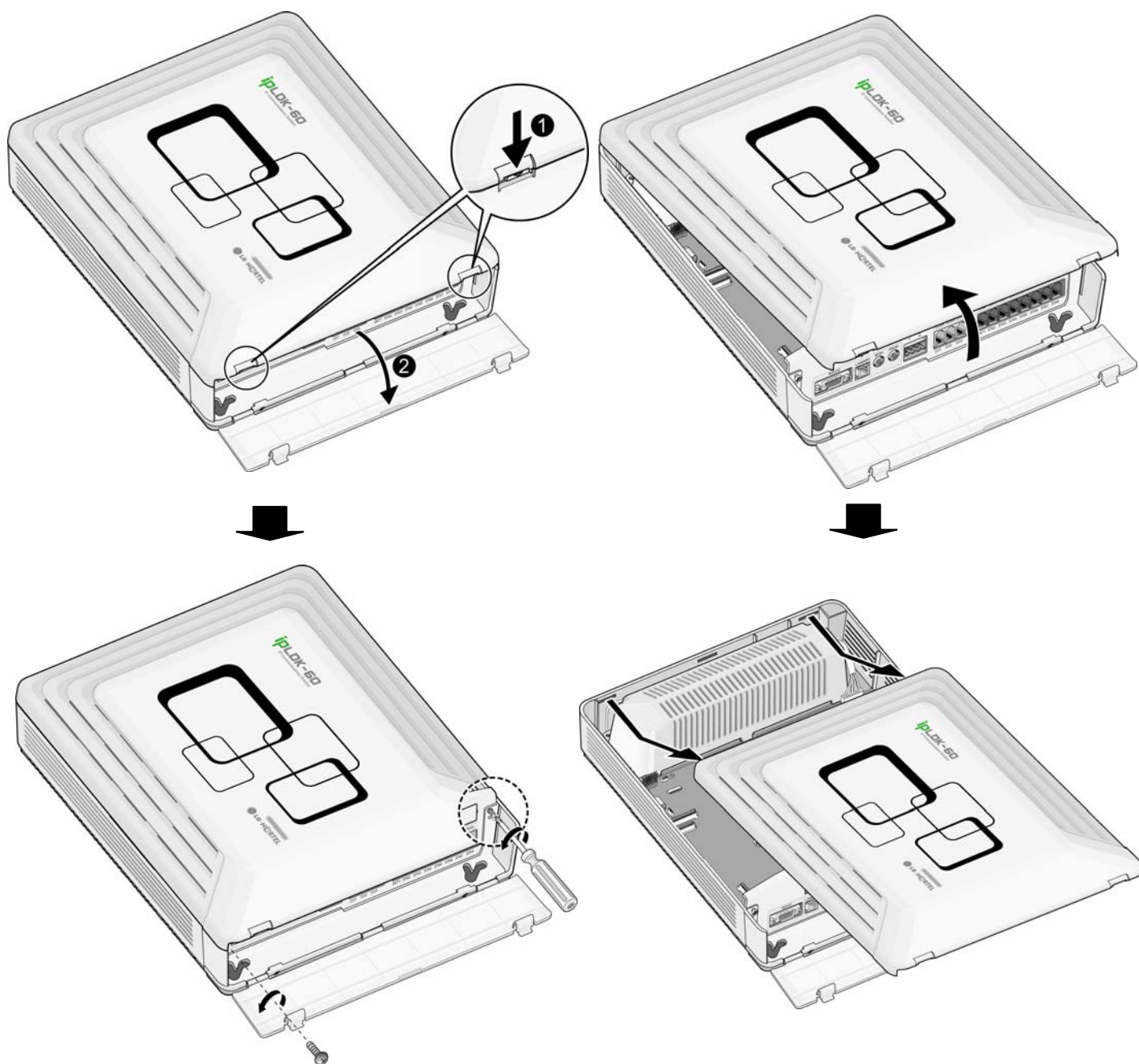
Рис. 3.2.3.1 Снятие лицевой панели
