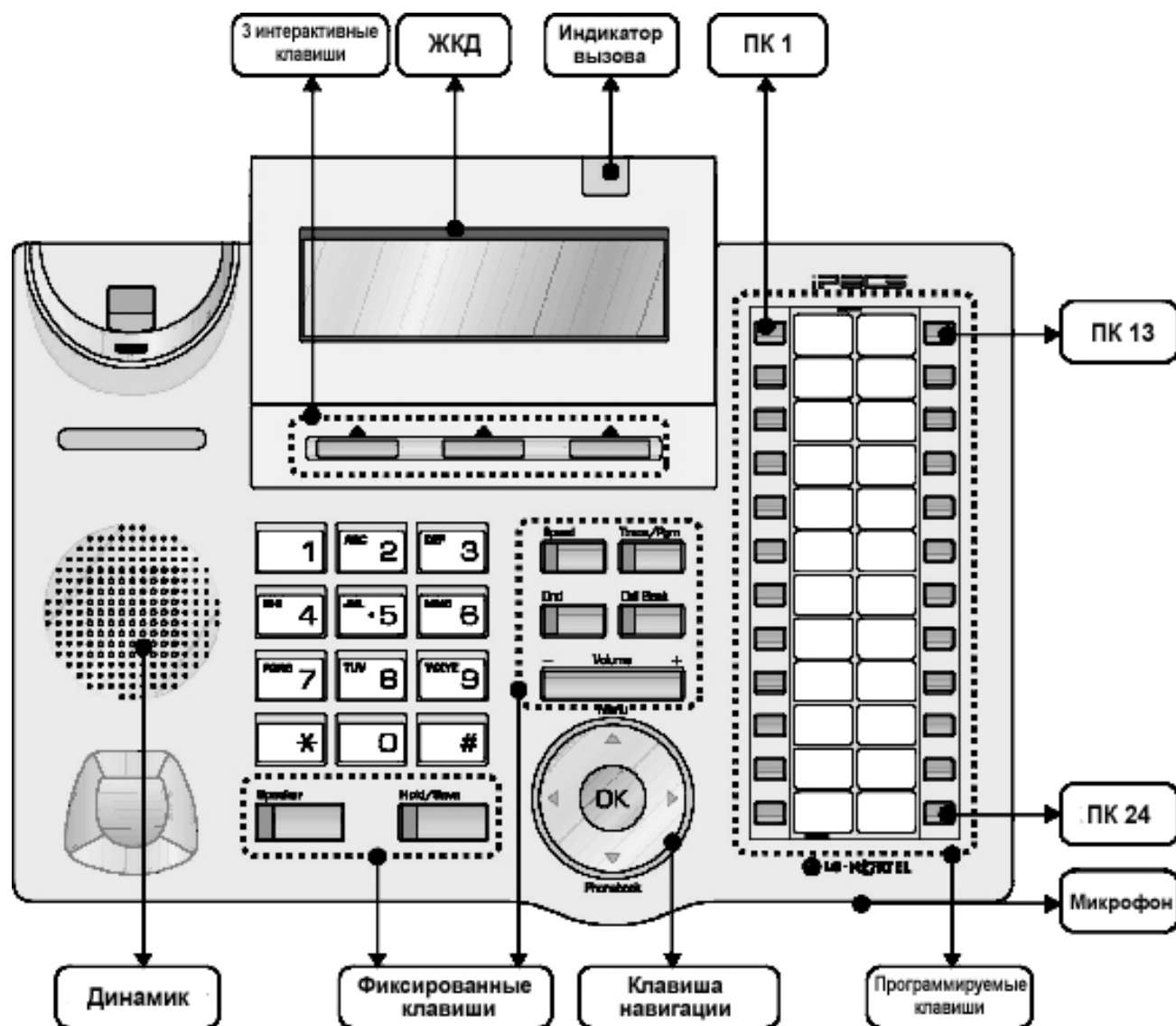
Рис. 6.2.1.2 Описание клавиш IP телефона LIP-7024D
