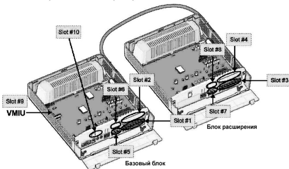
Рис. 6.2.3.2 Расположение платомест
