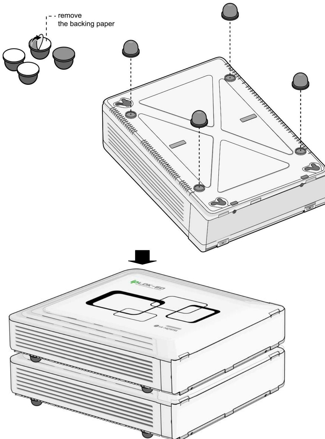
Рис. 3.2.7.3 Настольная / напольная установка
