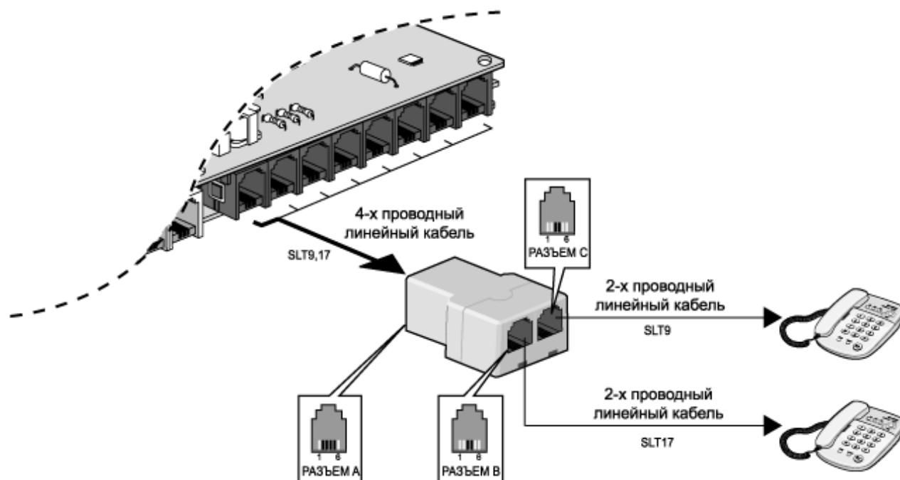
Рис. 4.4.2.2 Терминальный переходник
