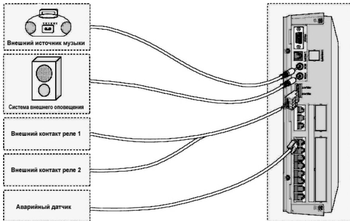
Рис. 5.1.3 Подключение дополнительных устройств
