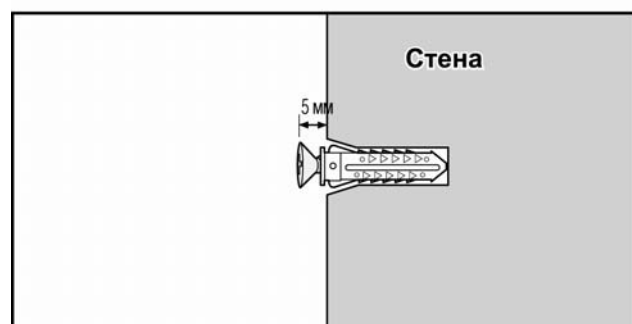
Рис. 3.2.7.1а Монтаж трафарета для настенного крепления
