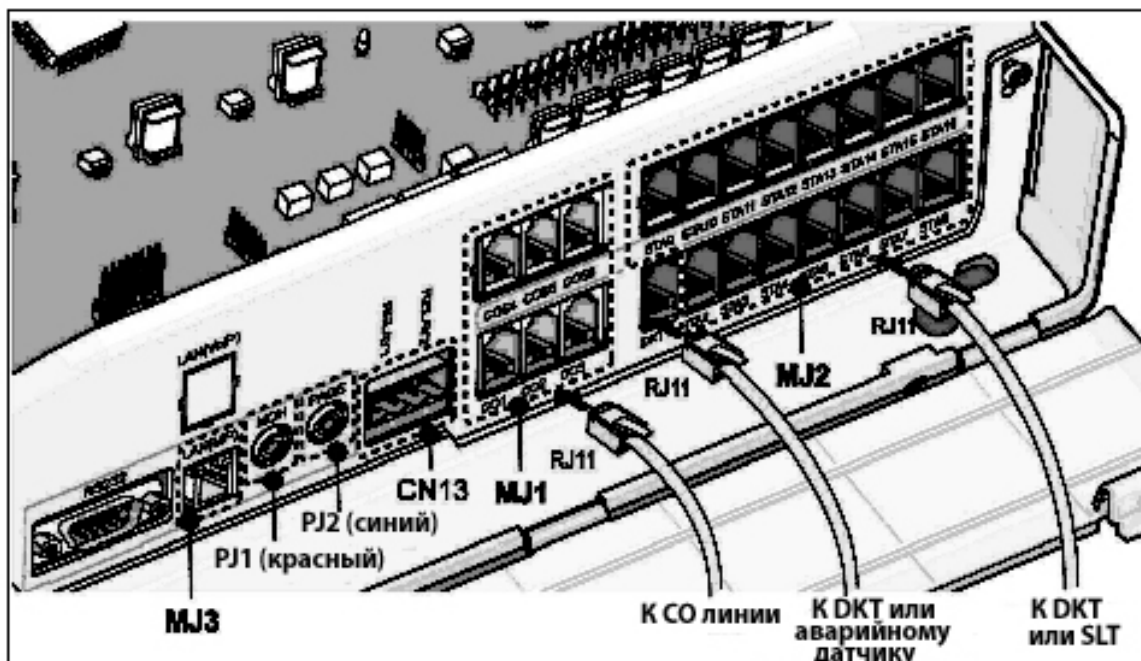
Рис. 4.26 Подключение по портам
